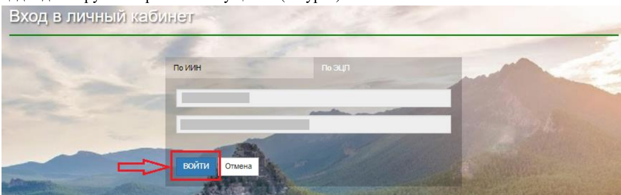
5-сурет. Авторизация
